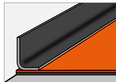
(3) Verzekeren de verbinding met de muren dankzij de zelfklevende randstrook
