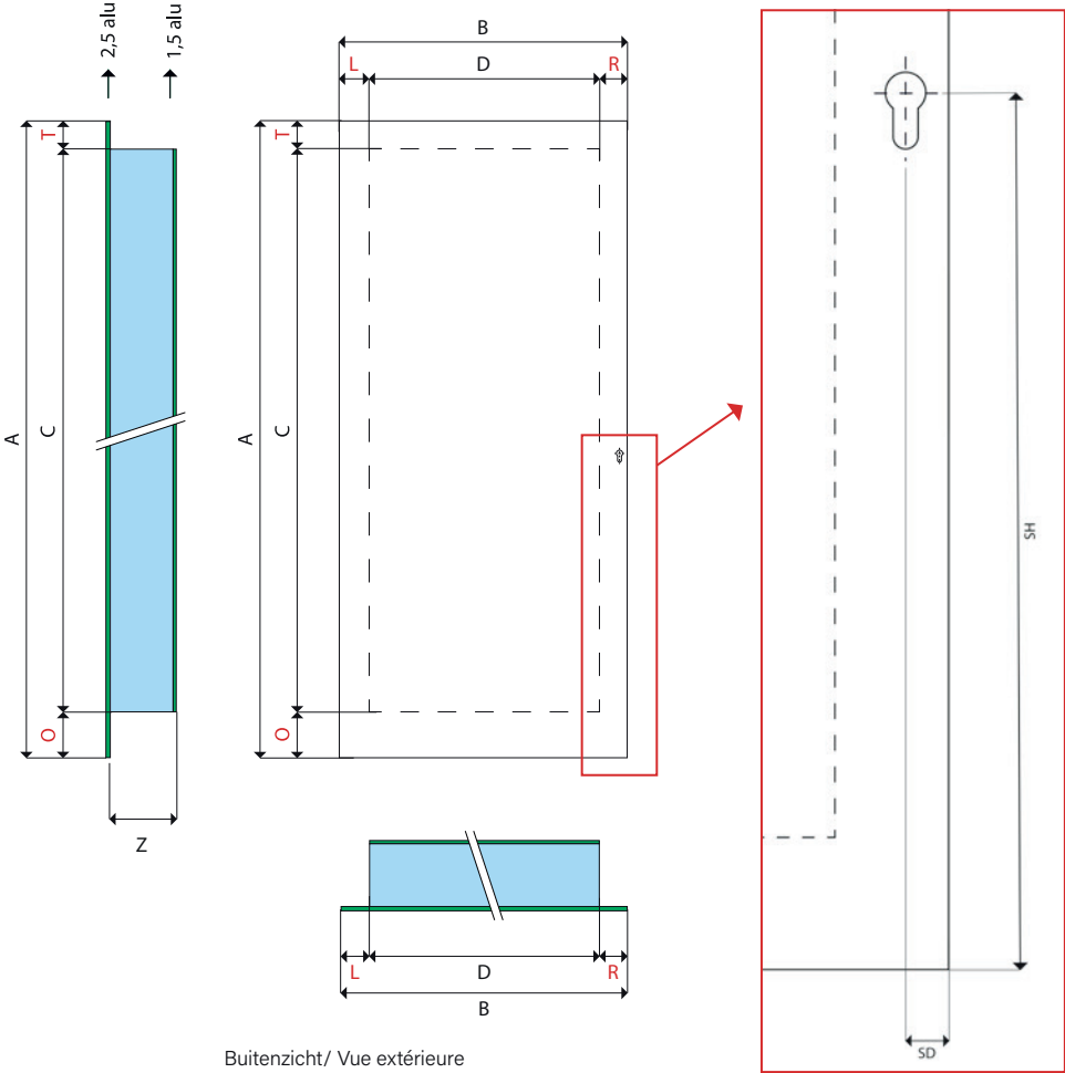
Buitenzicht/ Vue extérieure
